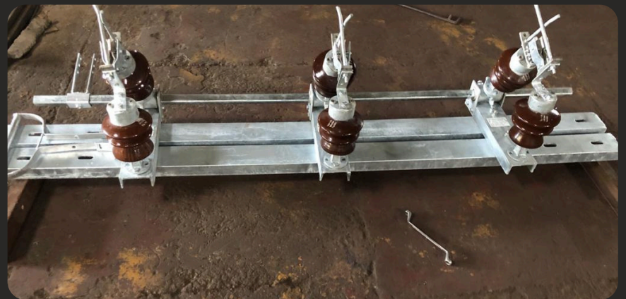
11 KV 400 Amp Porcelain AB Switch
